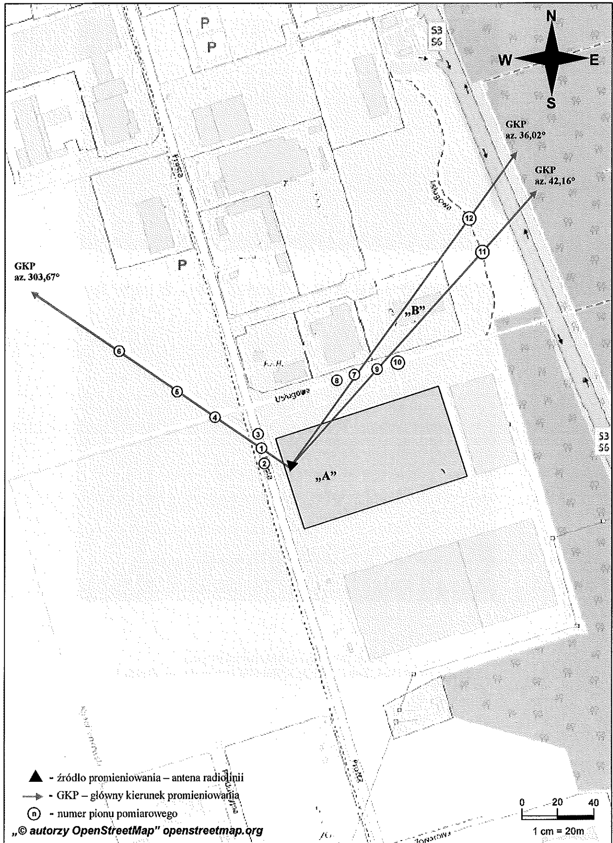
Rys. 1. Usytuowanie punktów i pionów pomiarowych w otoczeniu instalacji radiokomunikacyjnej Stacja Netia GOLNB017-GOLNM00008 Łozienica, ul. Prosta 16
