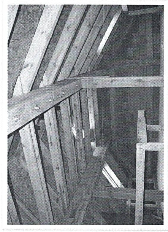
Konstrukcja drewniana budynku mieszkalnego
